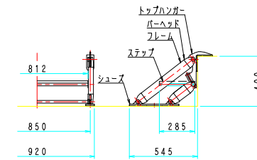
移動階段 FTR-400型
