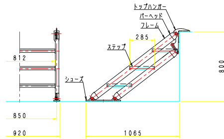
移動階段 FTR-800型
