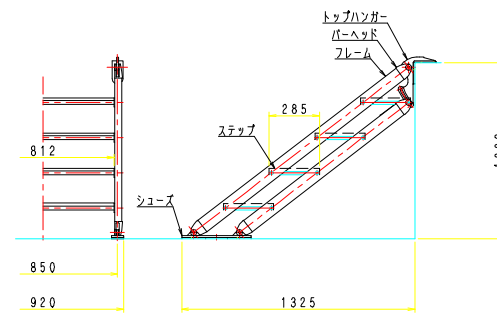
移動階段 FTR-1000型
