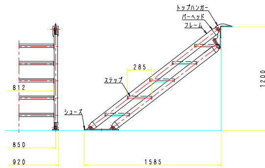
移動階段 FTR-1200型
