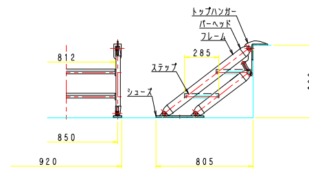
移動階段 FTR-600型
